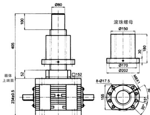
R:螺母升降
