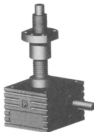
滚珠丝杠螺旋升降机
