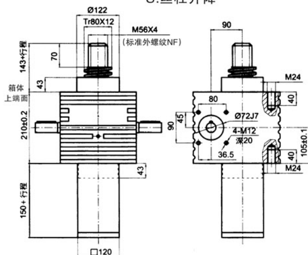
S:丝杠升降
